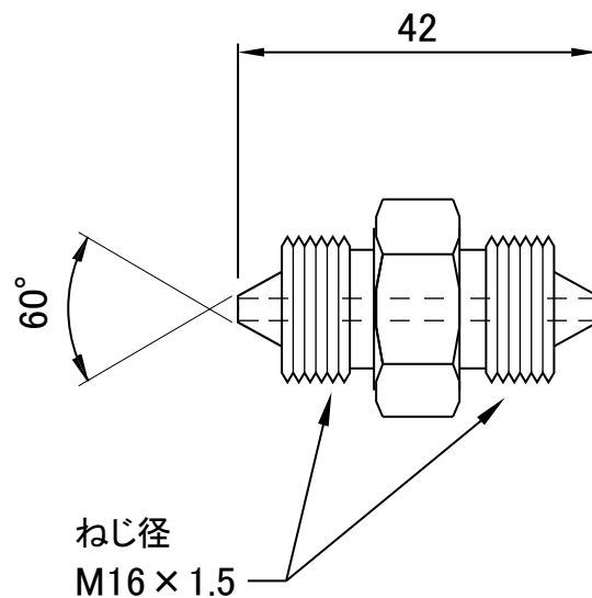
[ 高圧継手アダプター ]
